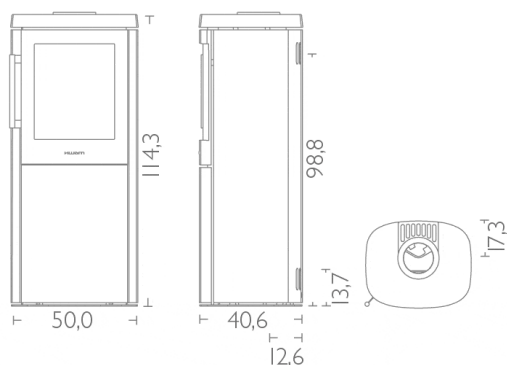
Rozměry HWAM 4540
