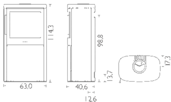
Rozměry HWAM 4640
